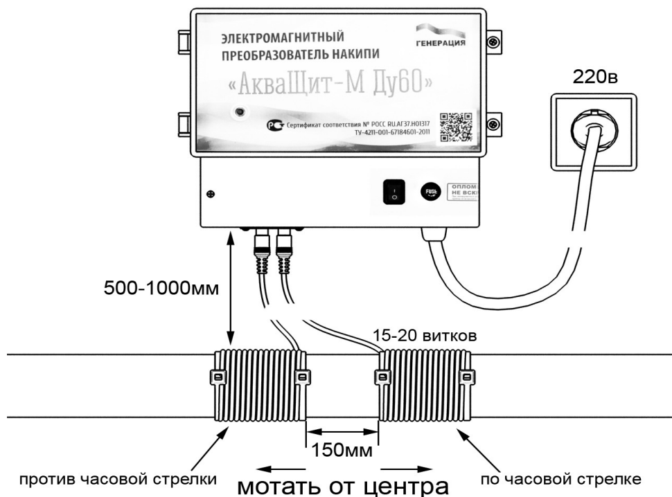
Рисунок 1. Условная схема монтажа прибора и проводов-излучателей
